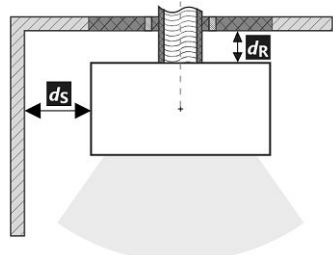
Hátsó kéménycsatlakozás (szigetelt)
