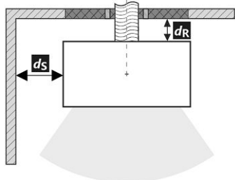
Tylne podłączenie przewodu kominowego
