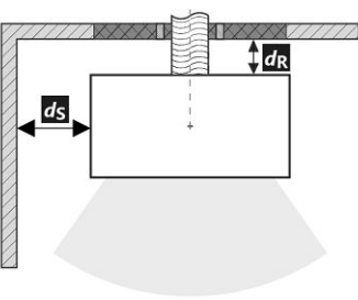
Подключение заднего дымохода
